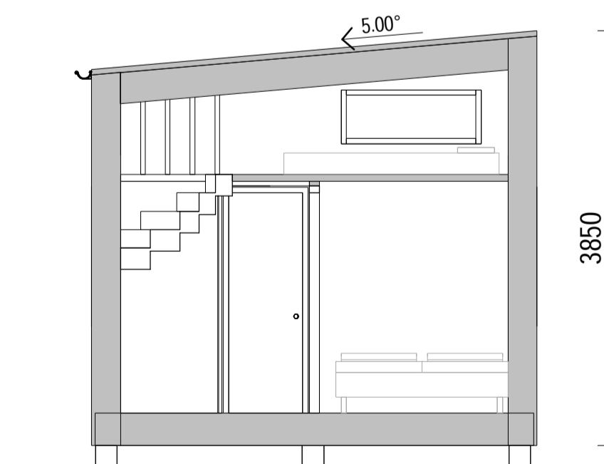
SEKTION A-A
